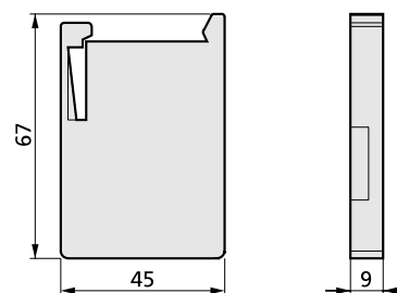
Spacer
